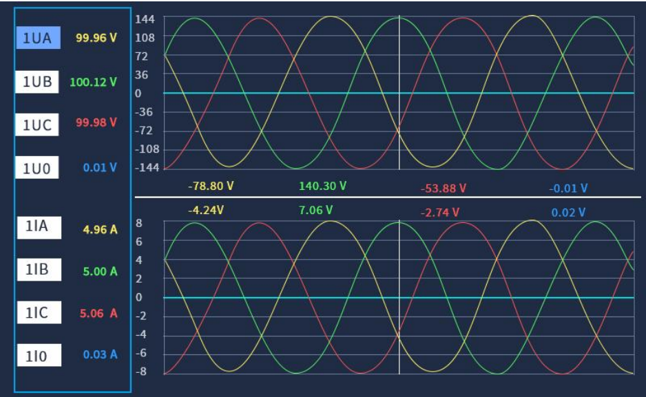
图4.7 实时波形
