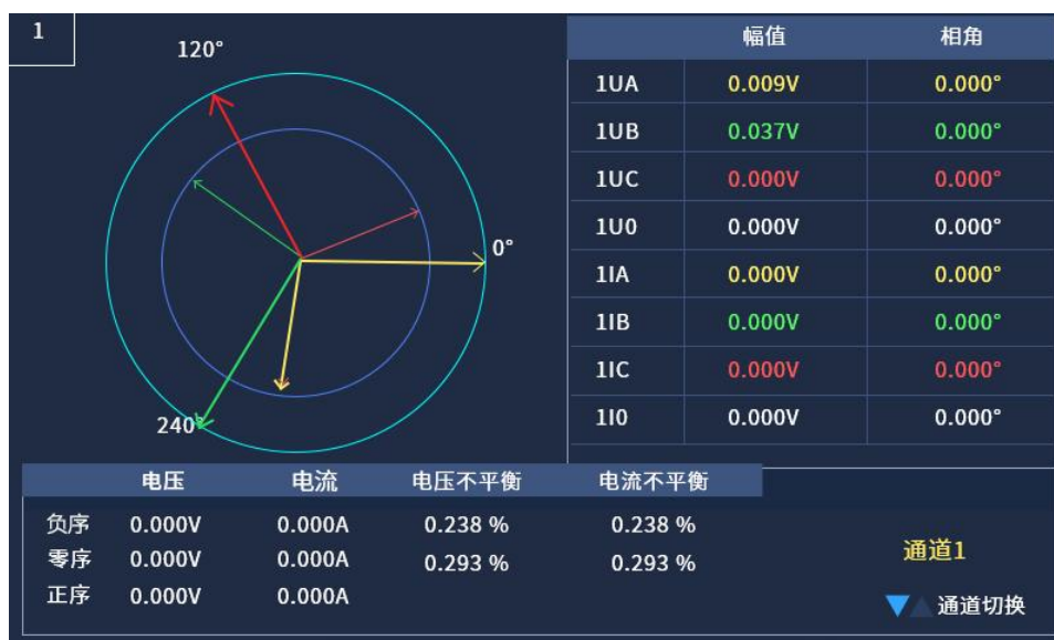
图4.8 矢量图
