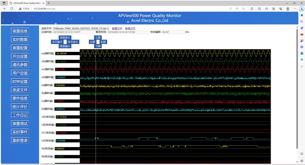
图 1.4 波形界面
