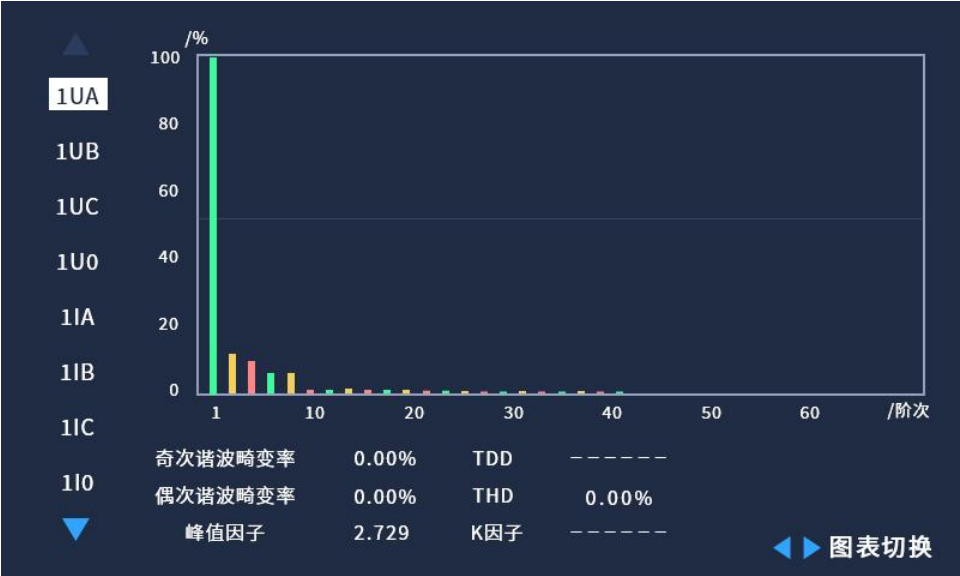
图 4.13 谐波柱状图
