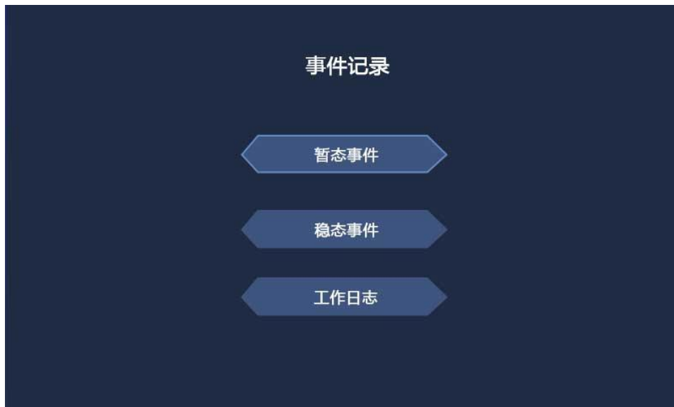
图 4.20 事件记录
