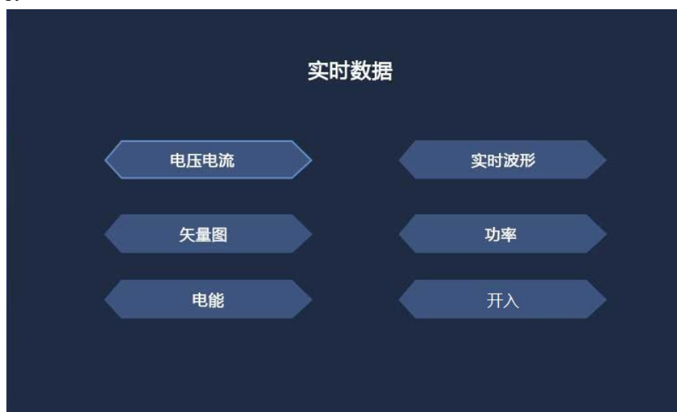
图4.5 实时数据
