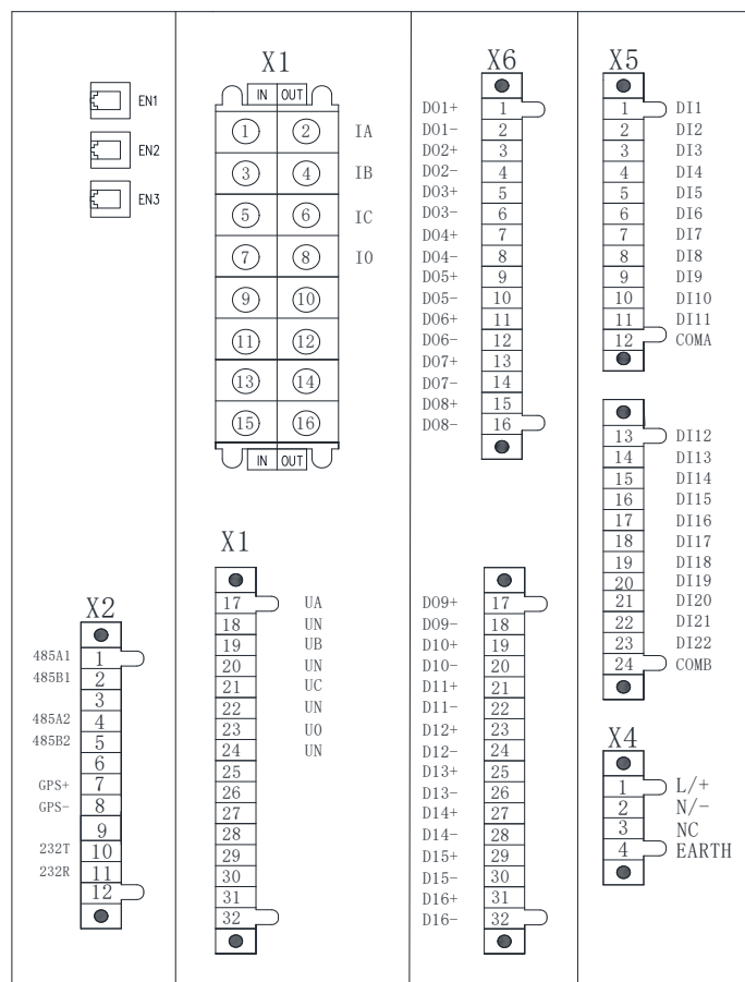
图 3.4 1U1I 背部端子图
