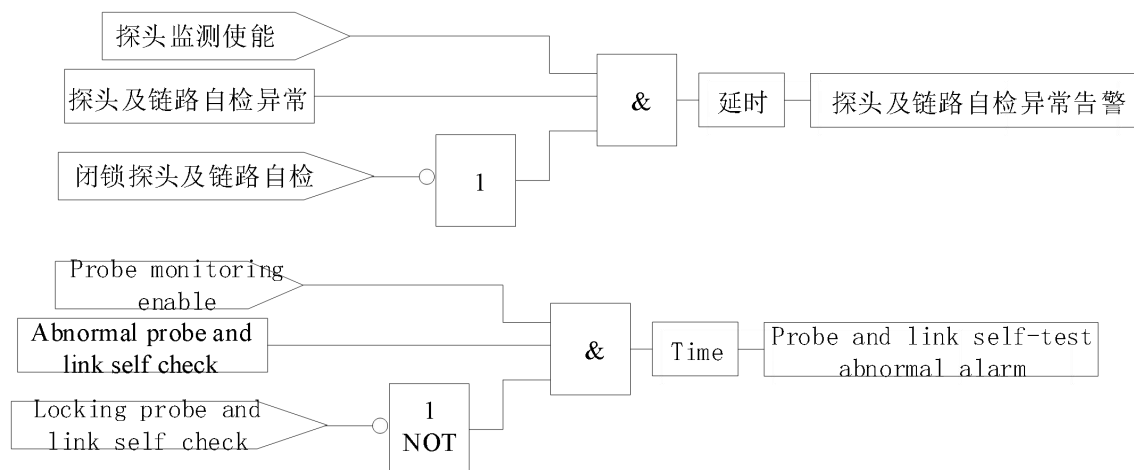
图 1.5 弧光传感器及光纤链路自检逻辑示意图
