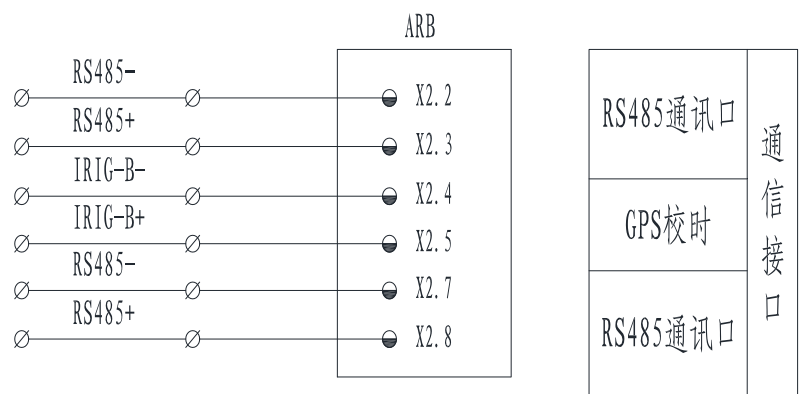
图 3.9 通信接口示意图
