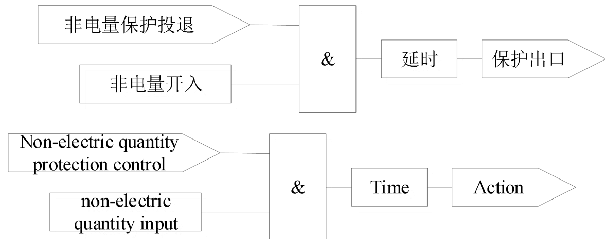
图 1.8 非电量保护逻辑示意图
