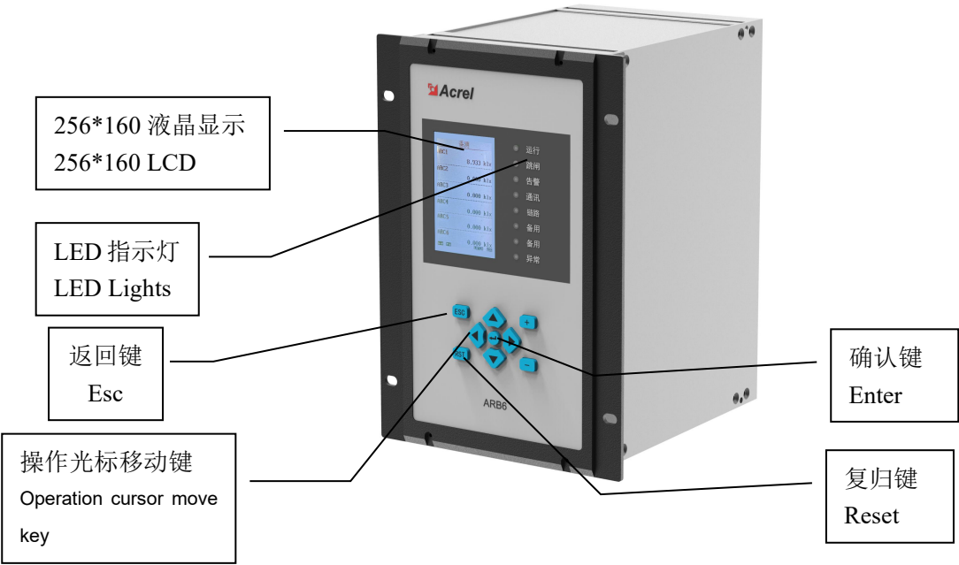
图 4.1 ARB6 前面板 Figure 4.1 ARB6 Front Panel
