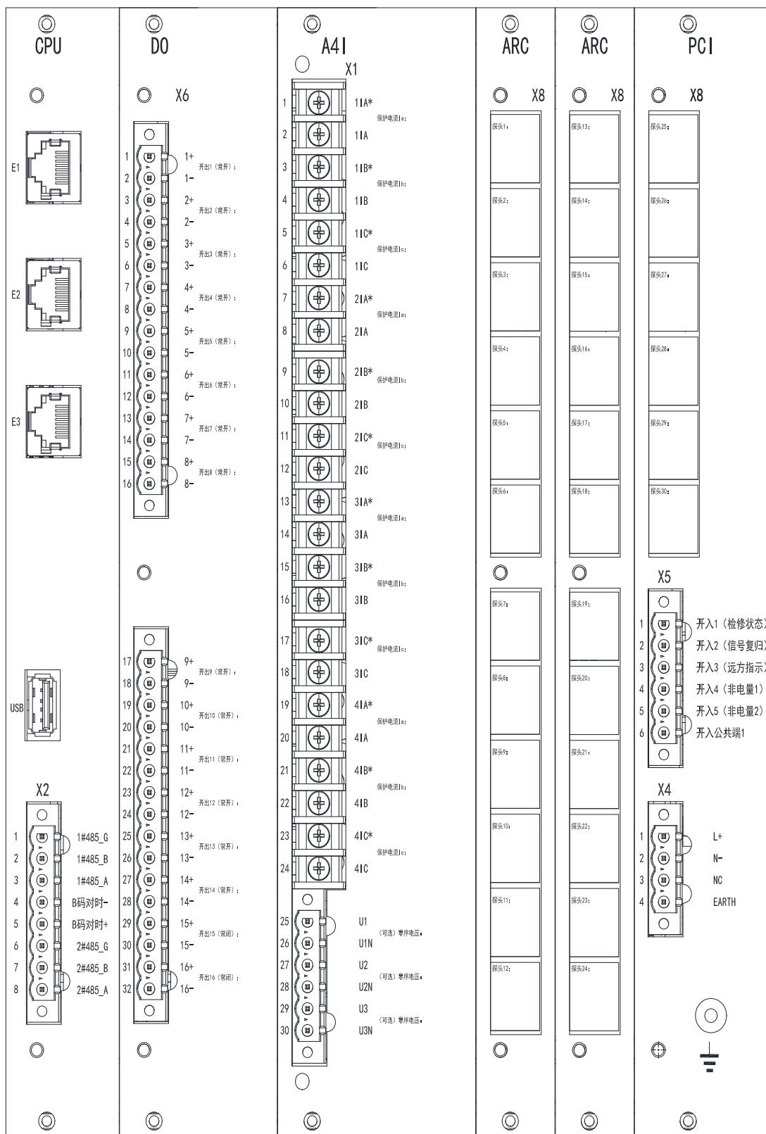
图 3.1 ARB6-A30 背板端子定义图 Figure 3.1 ARB6-A30 Backplane Diagram
