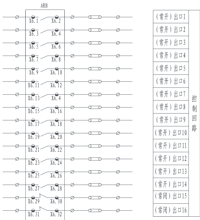
图 3.8 控制回路二次原理图
