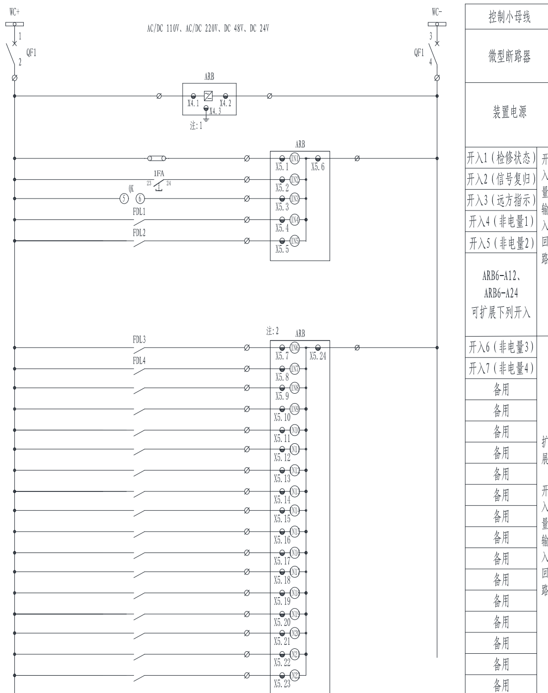
图 3.7 装置电源、开入量回路二次原理图
