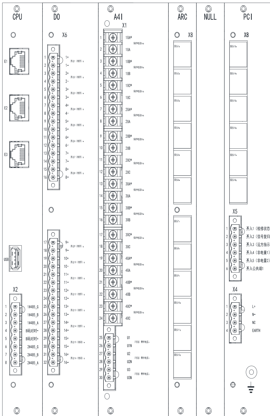
图 3.3 ARB6-A18 背板端子定义图
