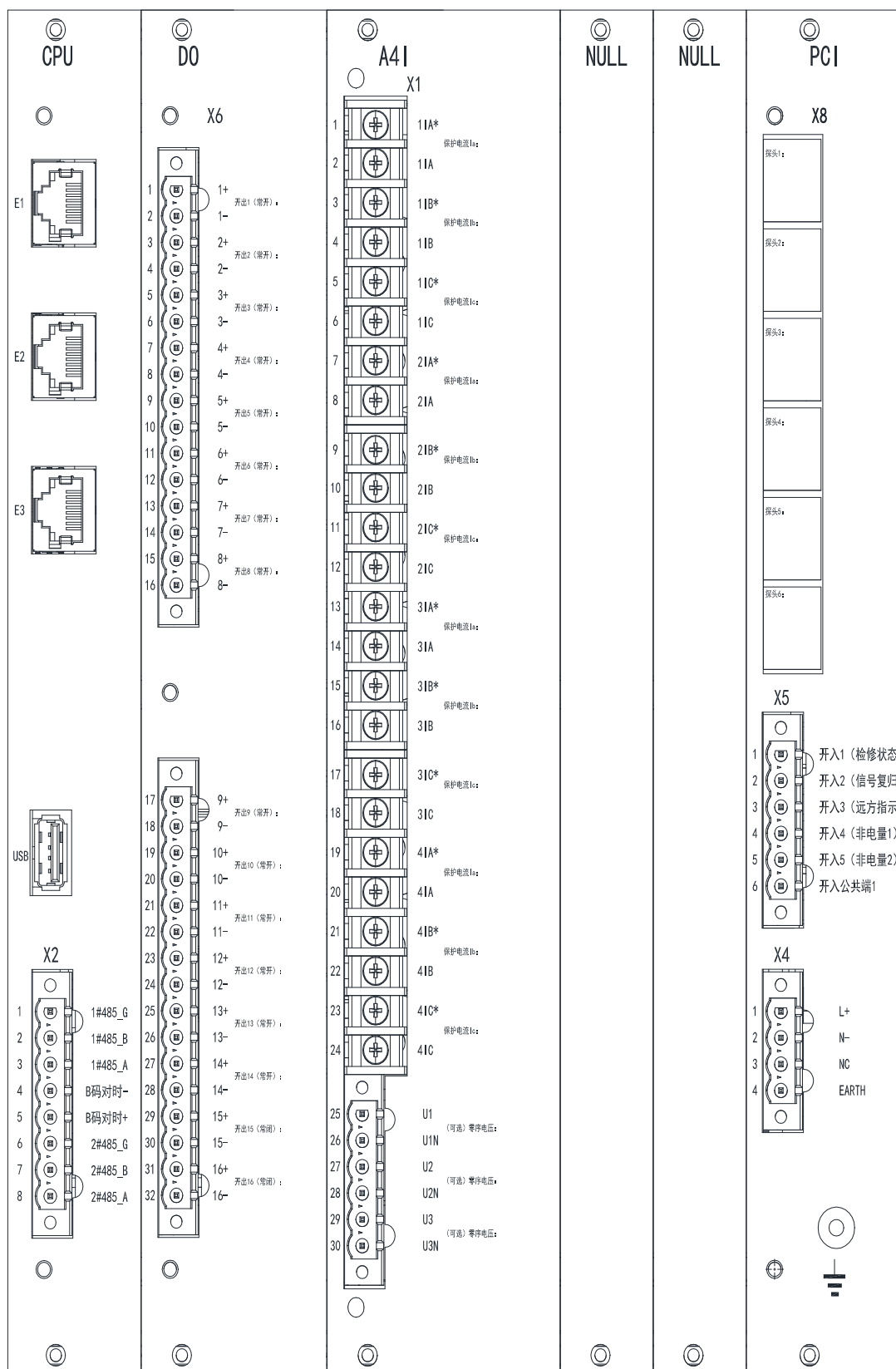
图 3.5 ARB6-A6 背板端子定义图 Figure 3.5 ARB6-A6 Backplane Diagram
