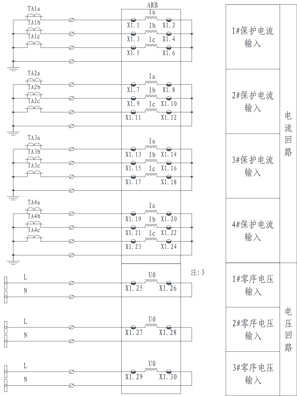
图 3.6 电流、电压回路二次原理图
