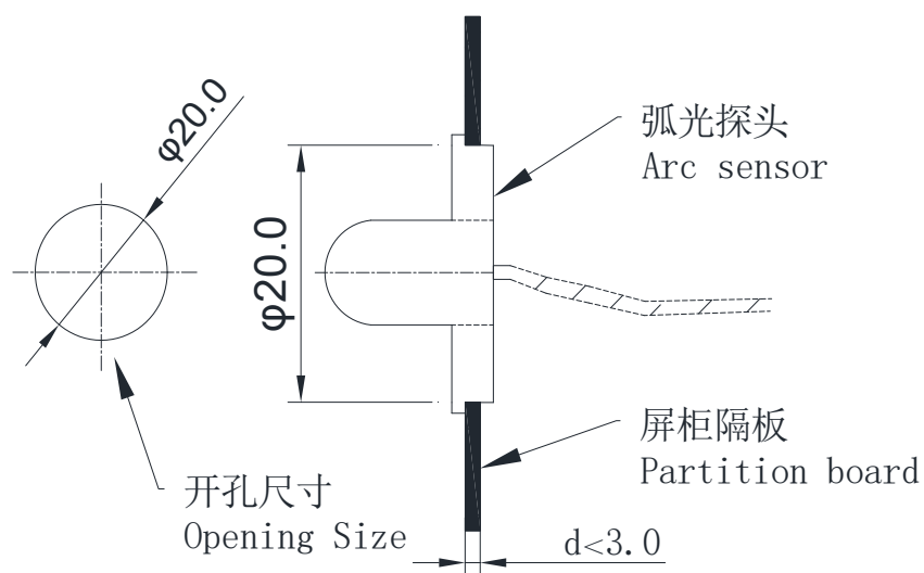
图 3.4 弧光传感器外形及开孔尺寸图
