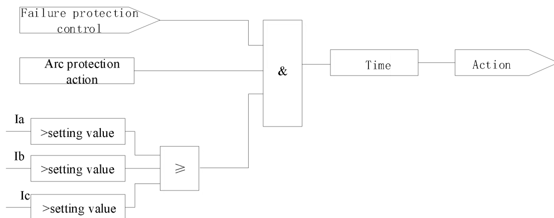
图 1.6 失灵保护逻辑示意图
