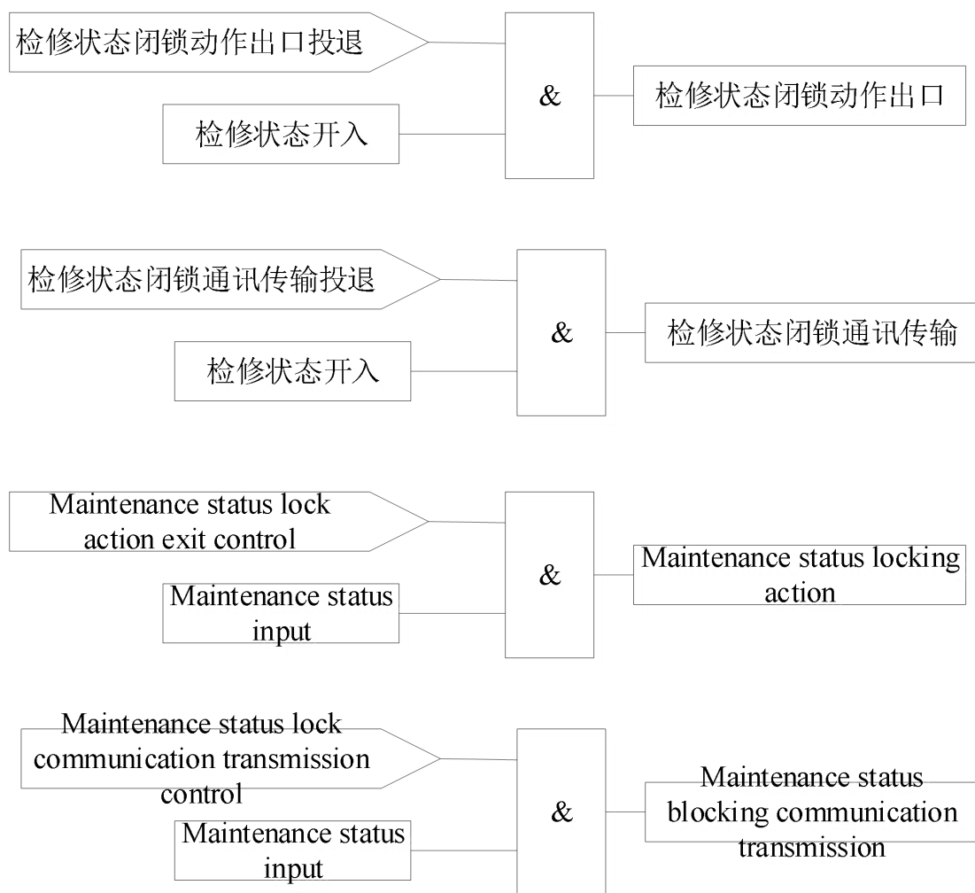
图 1.9 检修状态闭锁逻辑示意图
