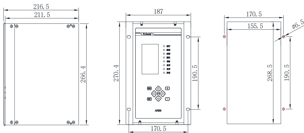
图 3.2 弧光保护装置外形及开孔尺寸图
