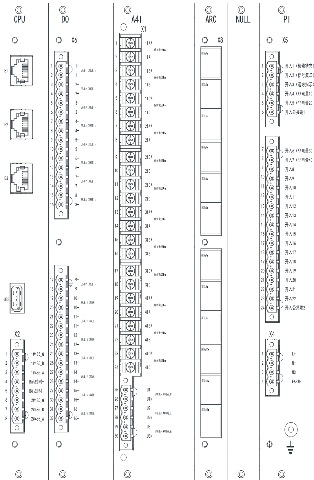
图 3.4 ARB6-A12 背板端子定义图 Figure 3.4 ARB6-A12 Backplane Diagram
