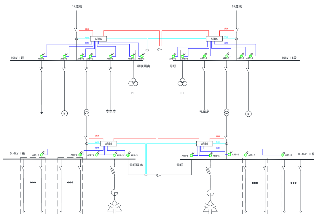
图 1.1 ARB6 母线弧光保护典型配置图
