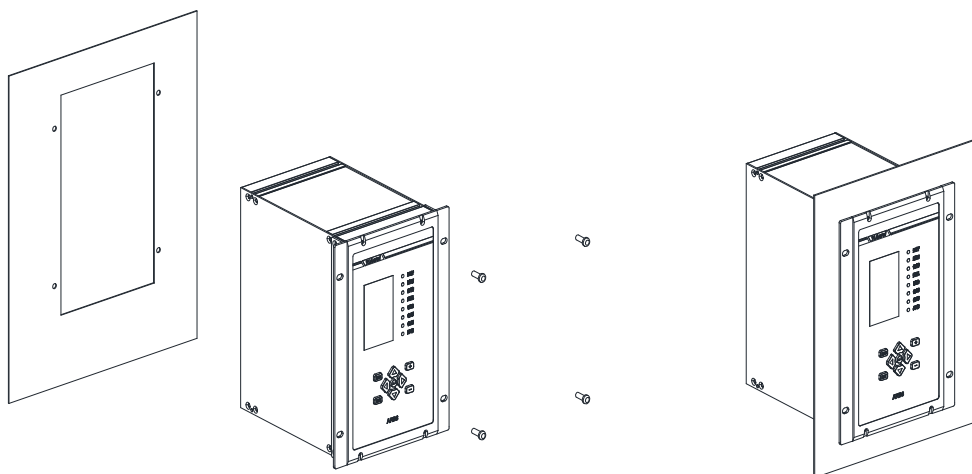
图 3.3 弧光保护装置安装示意图
