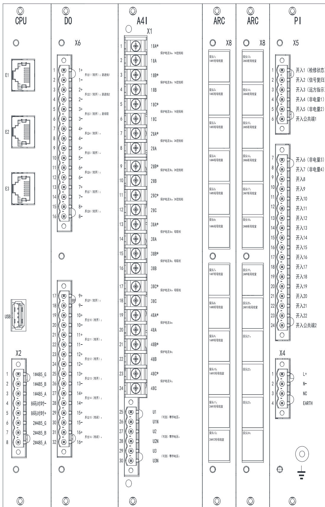
图 1.3 示例二背板端子接线示意图
