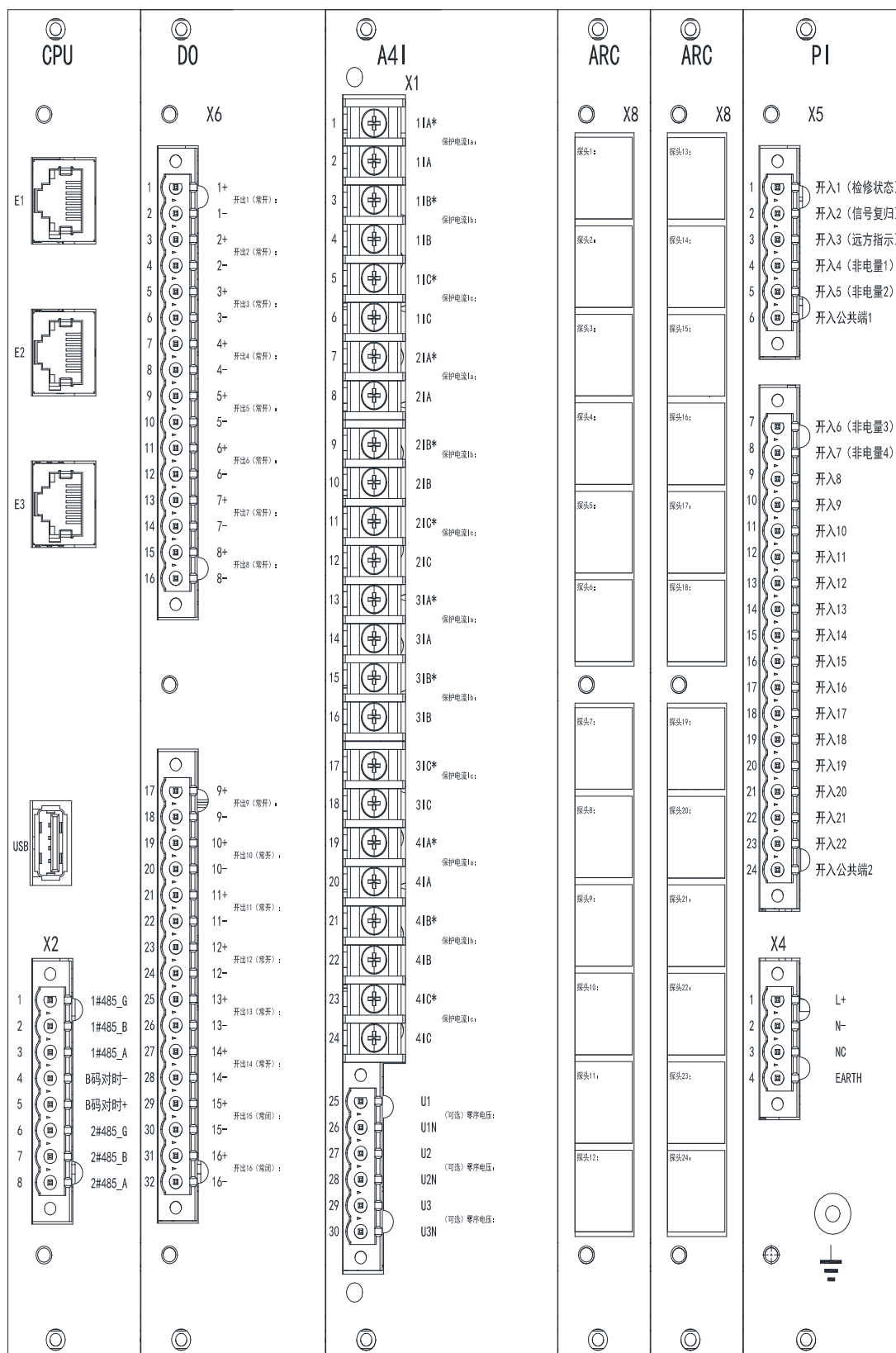
图 3.2 ARB6-A24 背板端子定义图 Figure 3.2 ARB6-A24 Backplane Diagram
