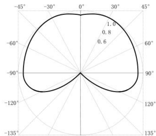
图 3.2 ARB-S1 弧光传感器监测范围角度
