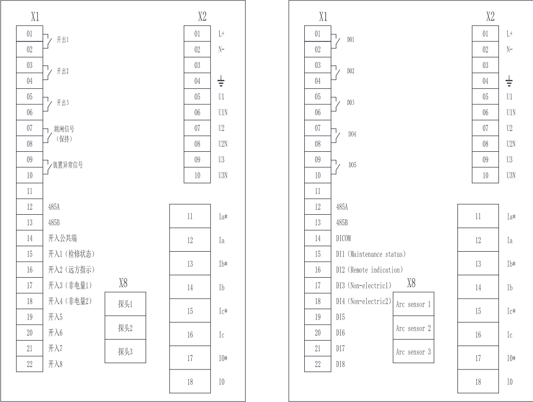
图 3.1 ARB4 背板端子定义图 Figure 3.1 ARB4 Backplane Diagram
