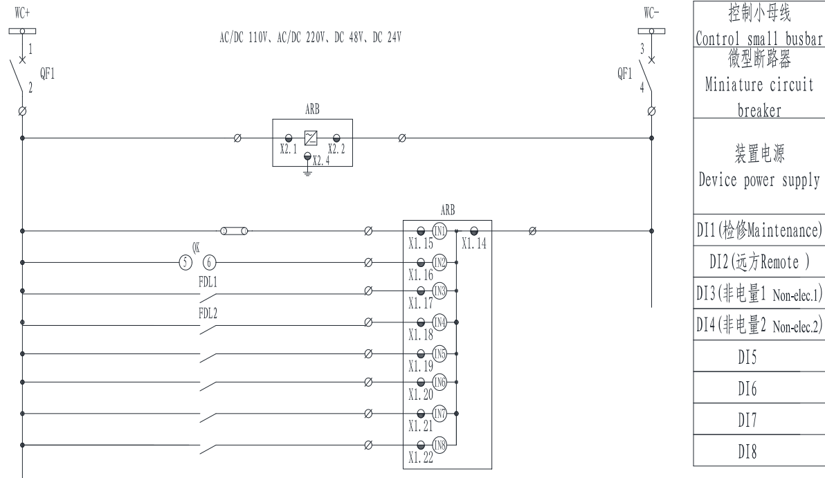
图 3.3 装置电源、开入量回路二次原理图
