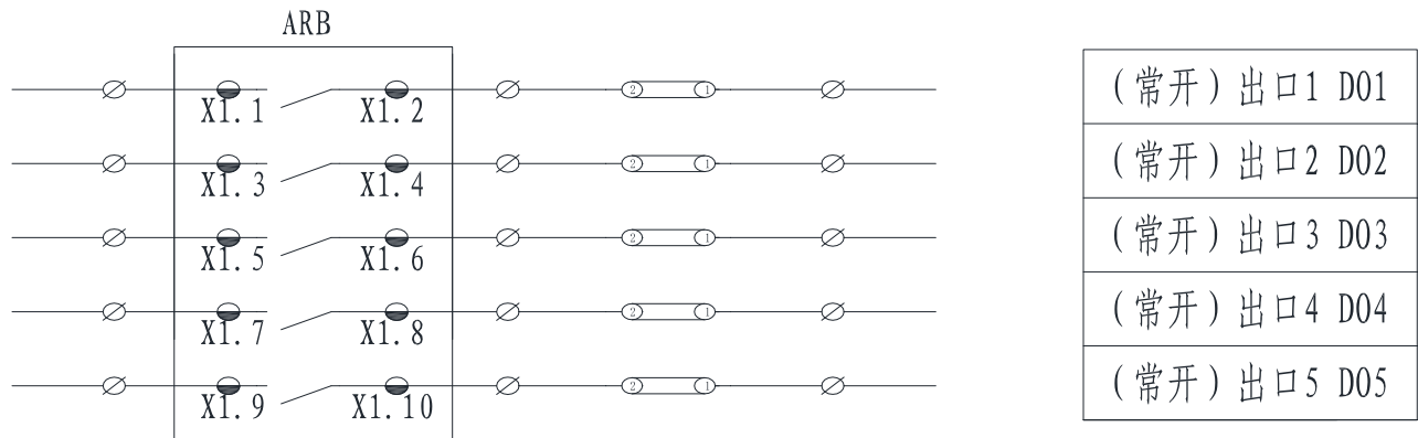
图 3.4 控制回路二次原理图
