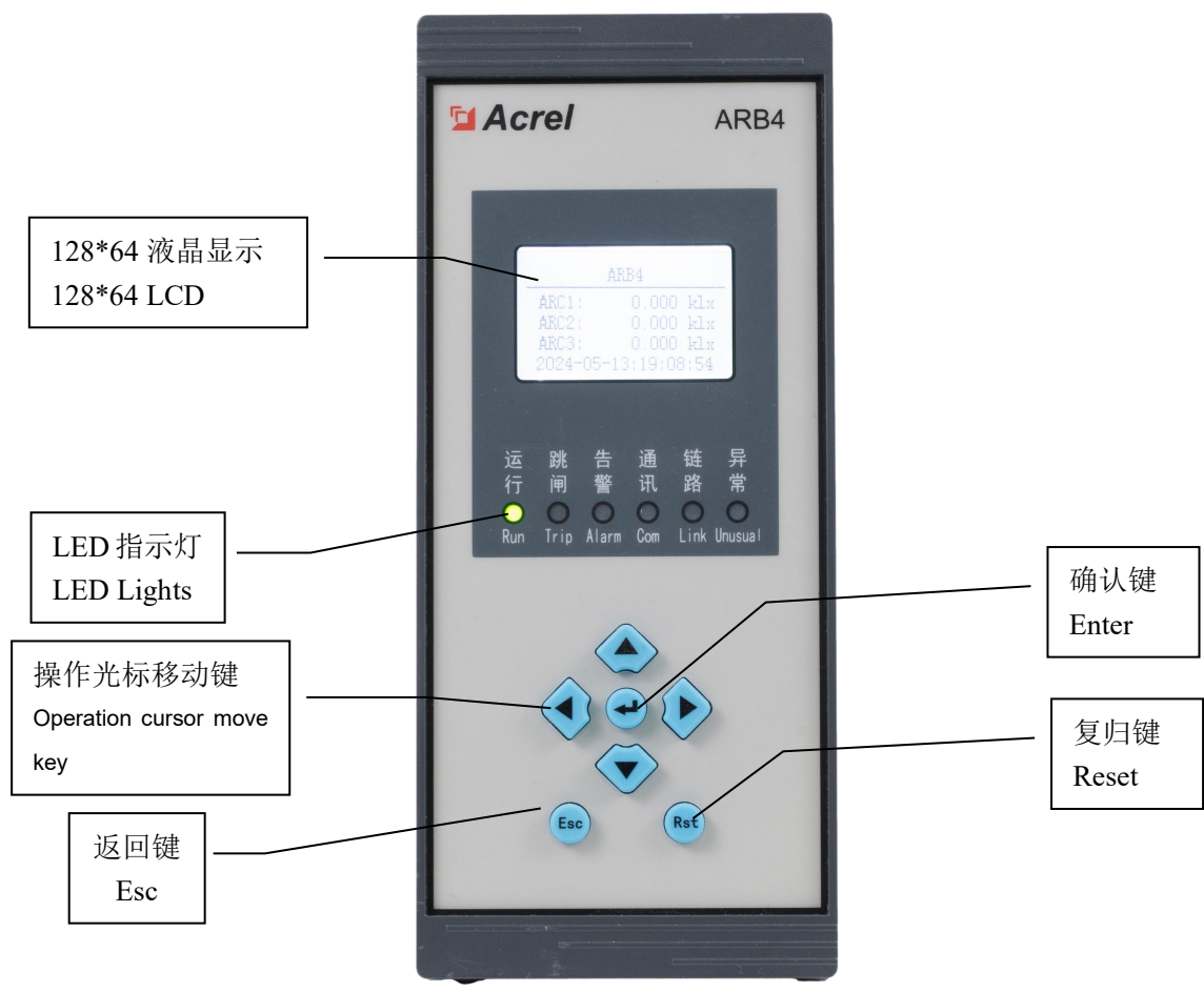
图 5.1 ARB4 前面板 Figure 5.1 ARB4 Front Panel
