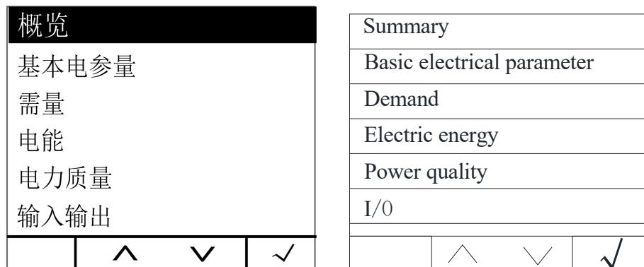
图 12 菜单界面
