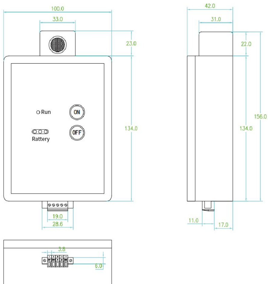
图 1.7 APD300-WP 尺寸图
