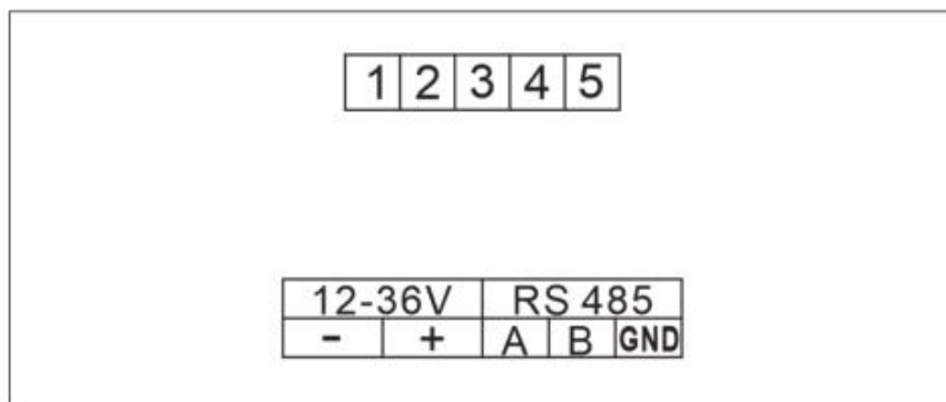
图 1.10 APD300-L 端子图
