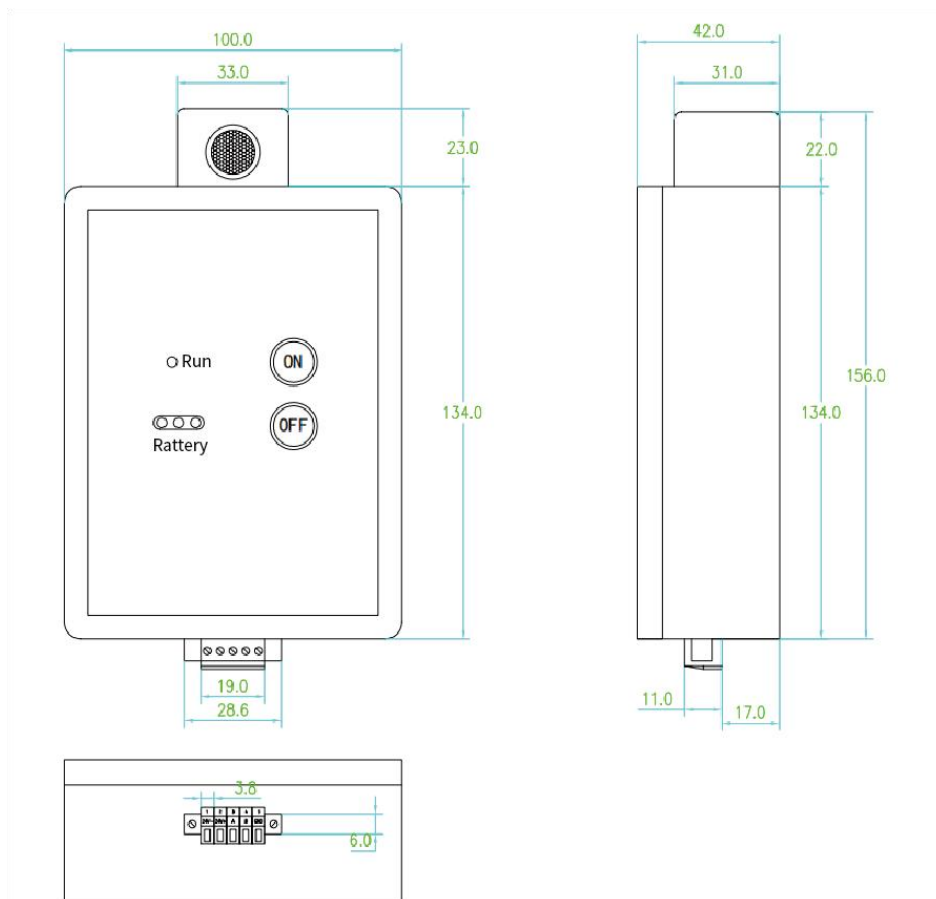
图 1.3 APD300-L 尺寸图
