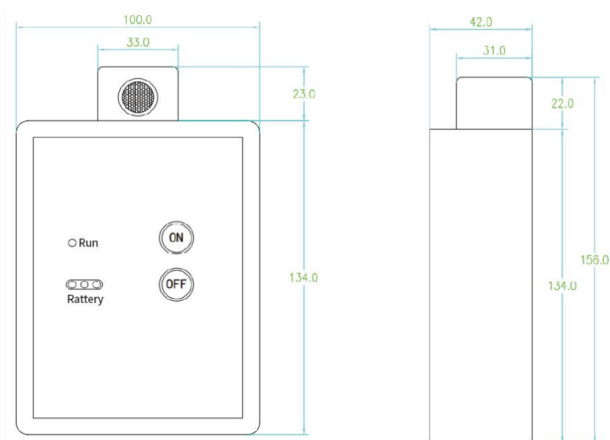
图 1.5 APD300-W 尺寸图
