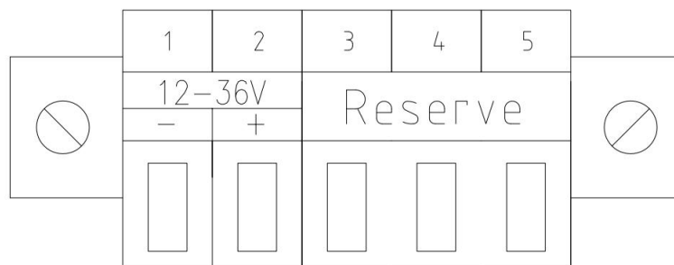
图 1.12 APD300-WP 端子图
