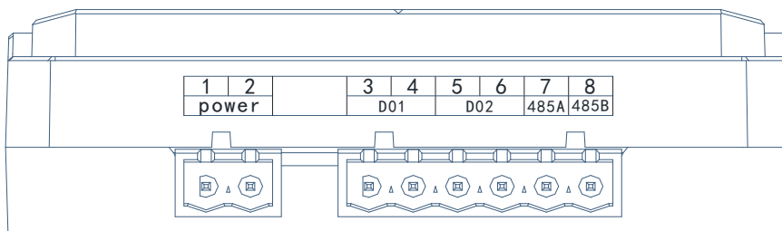
图 1.13 ATC600 端子图 Figure 1.13 ATC600 terminal diagram
