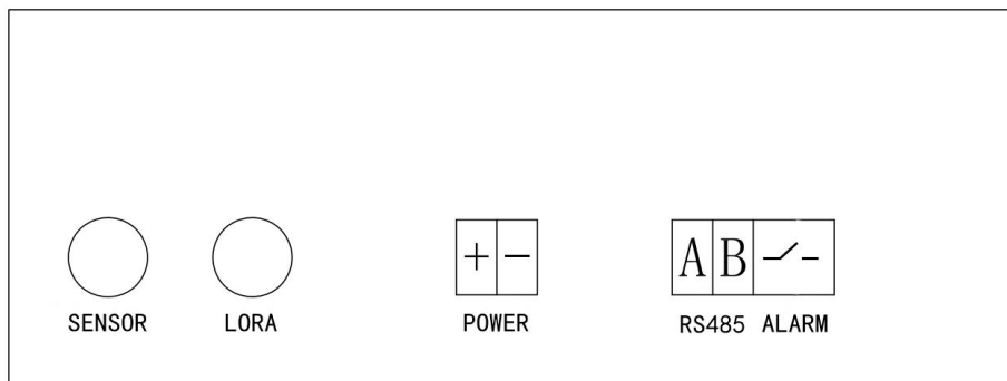
图 1.9 APD100 端子图
