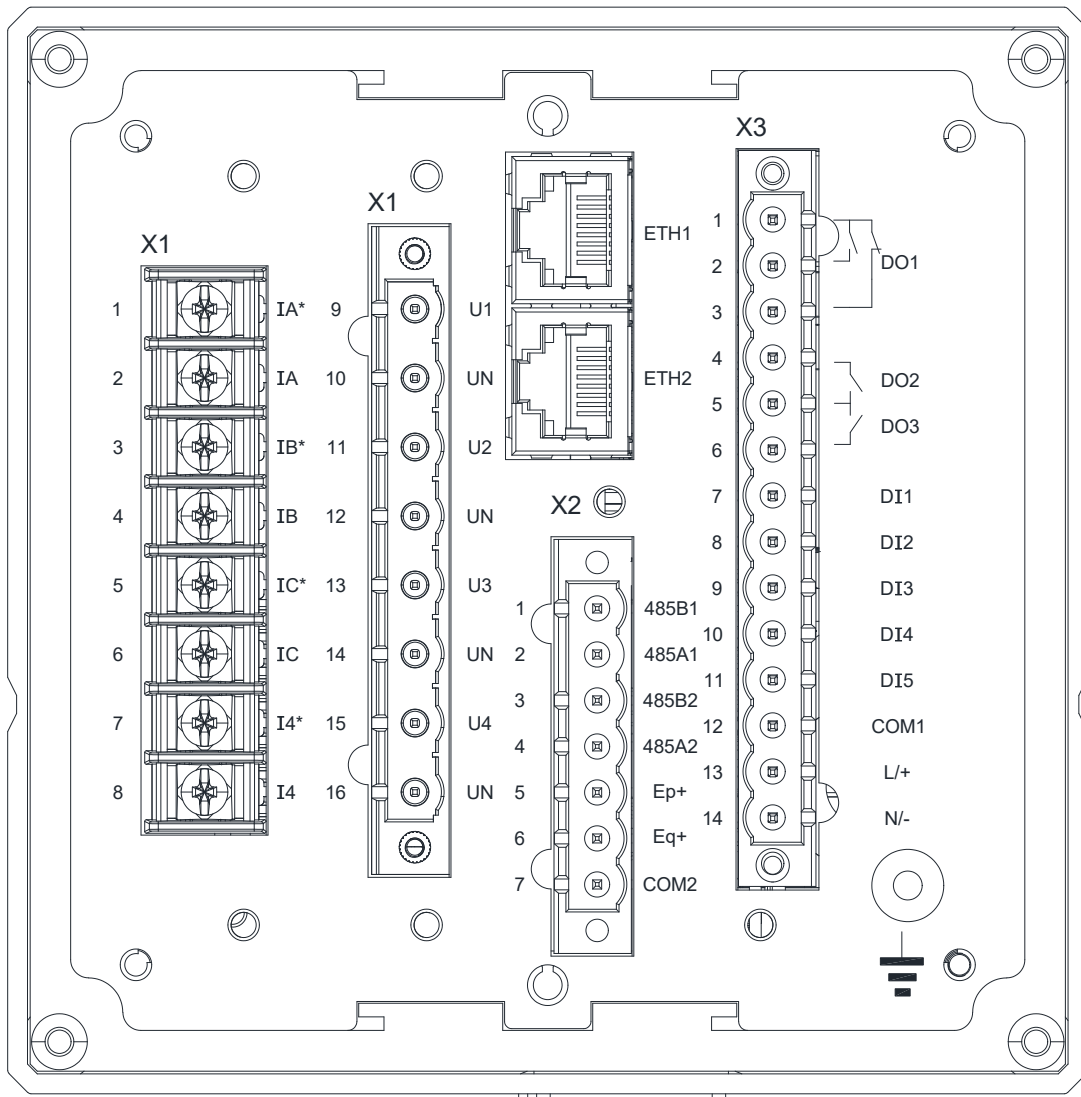
图 3.3 背部端子图
