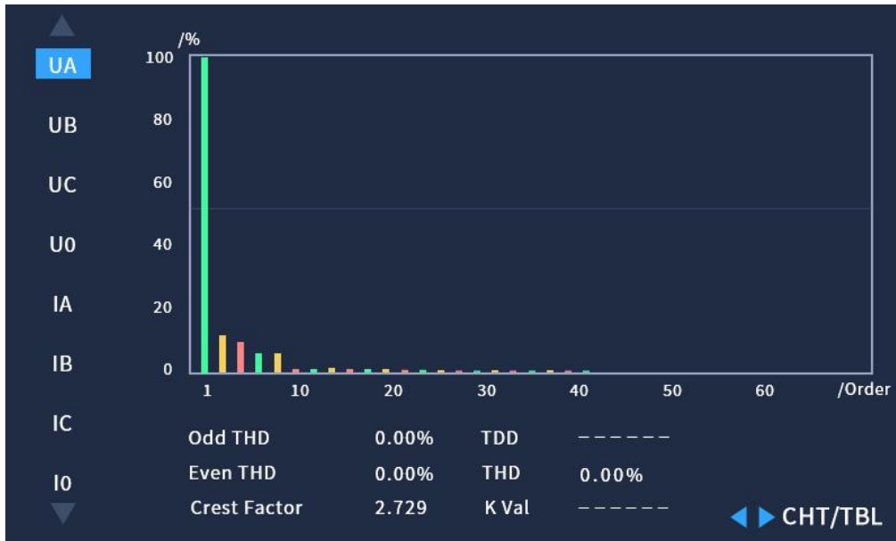
图 4.15 谐波柱状图
