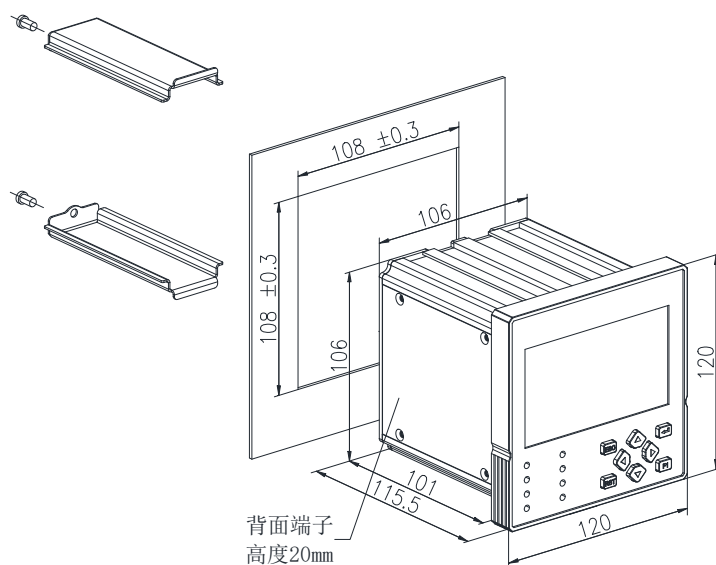
图 3.2 安装示意图
