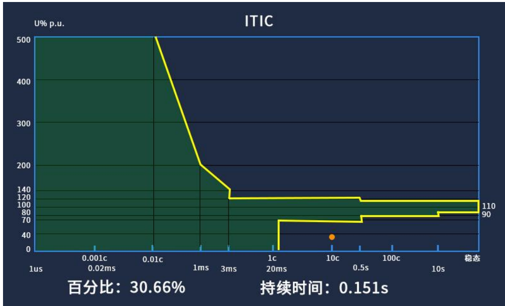
图 4.28(a) ITIC 容忍度曲线
